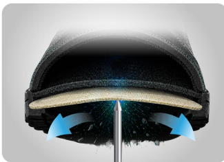
FlexBarrier™ Semelle Kevlar (1100N) Protection flexible avec un confort optimisé.
